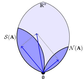
3.14. ábra: A lineáris algebra alaptétele: az A mátrix sortere és nulltere merőleges kiegészítő alterek. Eszerint a sortér bármely vektora merőleges a nulltér bármely vektorára, és \mathbb{R}^n bármely vektora egyértelműen felbomlik egy sortérbe és egy nulltérbe eső vektor összegére.
