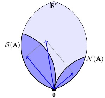
3.13. ábra: A lineáris algebra alaptétele: az A mátrix sortere és nulltere merőleges kiegészítő alterek. Eszerint bármely vektor, ami merőleges a nulltérre, a sortérben van. Ennek az is következménye, hogy \mathbb{R}^n bármely vektora egyértelműen felbomlik egy sortérbe és egy nulltérbe eső vektor összegére.
