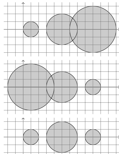
8.5. ábra: A B mátrix sorösszeg és oszlopösszeg szerinti Gersgorin köröi és ezek metszete. Utóbbi mutatja, hogy B -nek három valós sajátértéke van.
