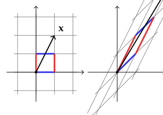
7.5. ábra: Az \mathbf{A} = \begin{bmatrix} 1 & 1 \\ 1 & 2 \end{bmatrix} mátrix hatása az egységnégyzetrácson, és az \mathbf{x} = (1, 2) vektoron. Az \mathbf{Ax} vektor végpontja a paralelogrammarácson 1 lépés az x -tengely képének irányába, és 2 lépés az y -tengely képének irányába.
